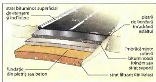
Elementele unui drum asfaltat modern
