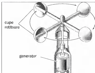
Anemometru electric cu palete în formă de cupă
