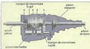
Transmisia la patru viteze, prin cutie cu schimbător manual. Arborele primar, în mișcare, rotește arborele intermediar, prin care se angrenează, pe rând, cele patru pinioane de mers înainte și pinionul marșarier de pe arborele de ieșire. Punerea în mișcare a arborelui de ieșire depinde de pinionul corespunzător vitezei alese cu ajutorul manșonului de sincronizare, manevrat de leverul schimbătorului de viteze (în cazul de față, este cuplat primul pinion). Pinioanele necuplate nu fac decât să se rotească în gol, fără să transmită putere.
