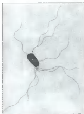
Bacteria Proteus vulgaris (la scară mare), prezentând filamente mobile (flageli)
