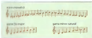
Exemple de guine: cromatică, majoră și minoră
