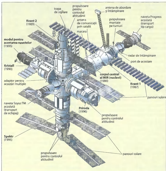
Stația spațială rusă/sovietică Mir, după îndeplinirea misiunii din 1996. Datele prezentate pentru fiecare modul reprezintă anul lansării sale. Andoate la stație sunt naveta cu echipaj uman Soyuz TM și naveta cargonă fără oameni la bord, pentru transportarea proviziilor
