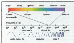
Spectru electromagnetic. Spectrul undelor electromagnetice se întinde de la undele radio de joasă frecvență la razele gamma de înaltă frecvență. Numai o mică porțiune din spectru este vizibilă ochiului uman, ea reprezentând lungimi de undă de oca 400–700 nanometri.
