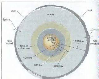
Secțiune transversală prin Lună, înfățișând asimetria în grosimea scoarței între fața vizibilă și invizibilă a Lunii și predominanța mărilor pe fața vizibilă. Distanțele indicate nu sunt la scară.
